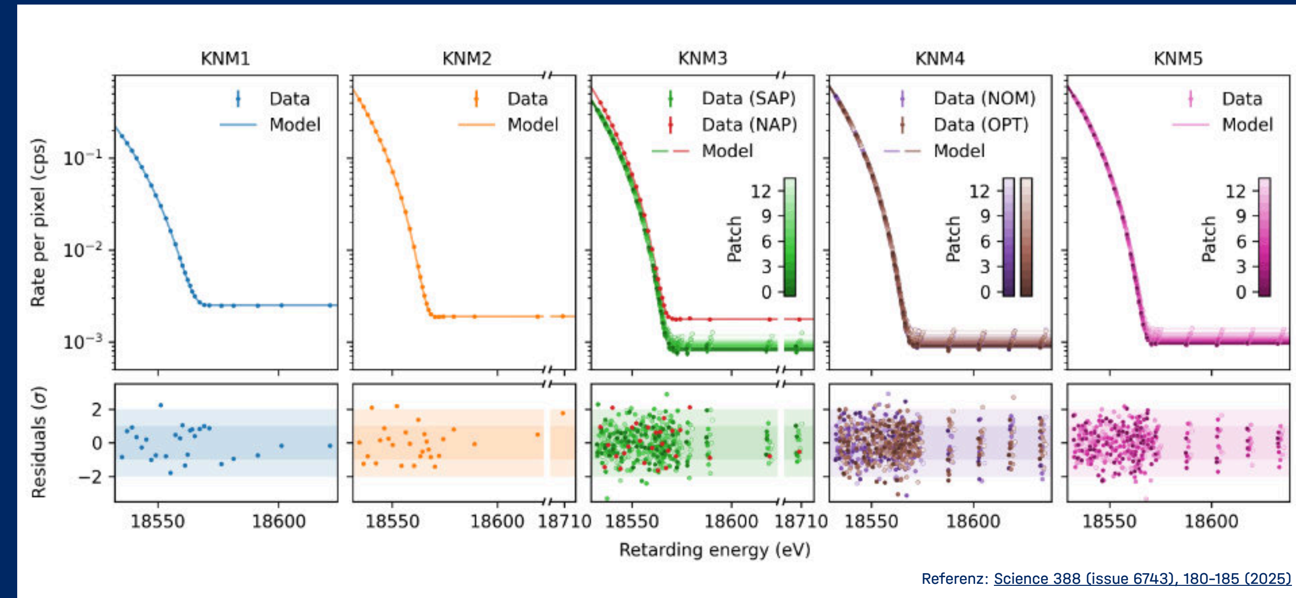
Präzisionsspektroskopie des Tritiumzerfalls mit den ersten fünf Runs der KATRIN-Messungen.
